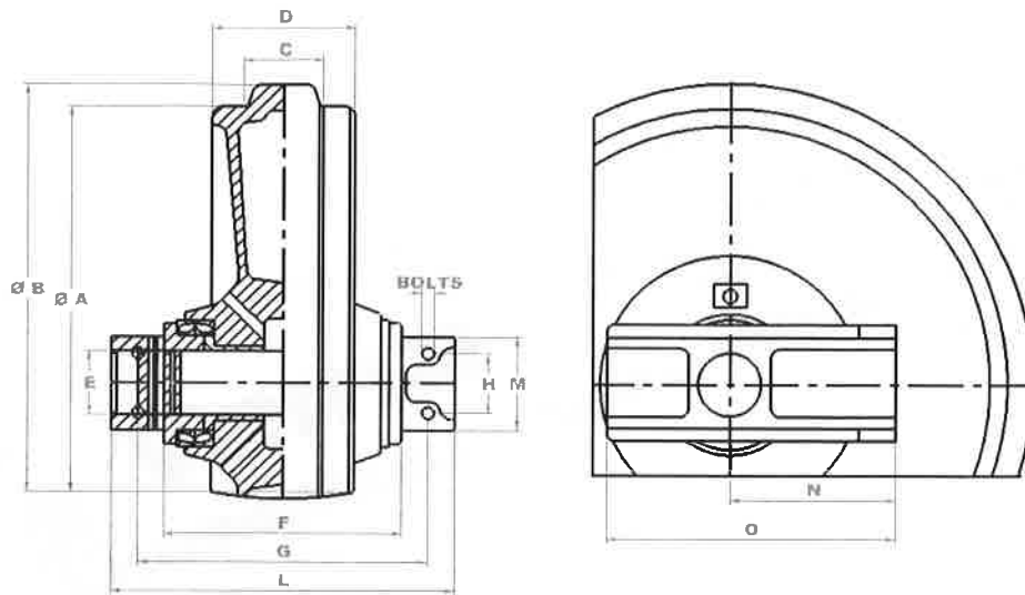
J01 Idler
