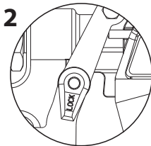
Gatilho desbloqueado (a pistola de pulverização pulveriza)
