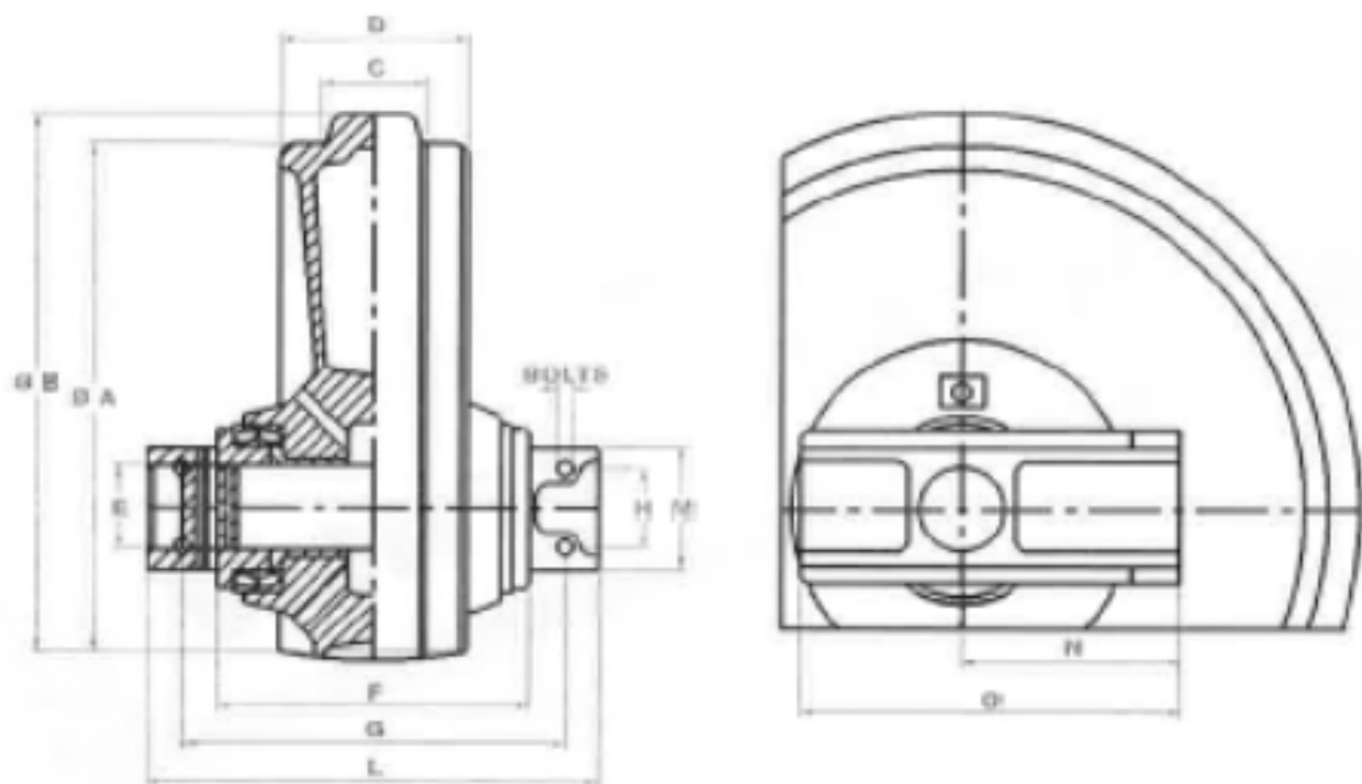
J01 Idler
