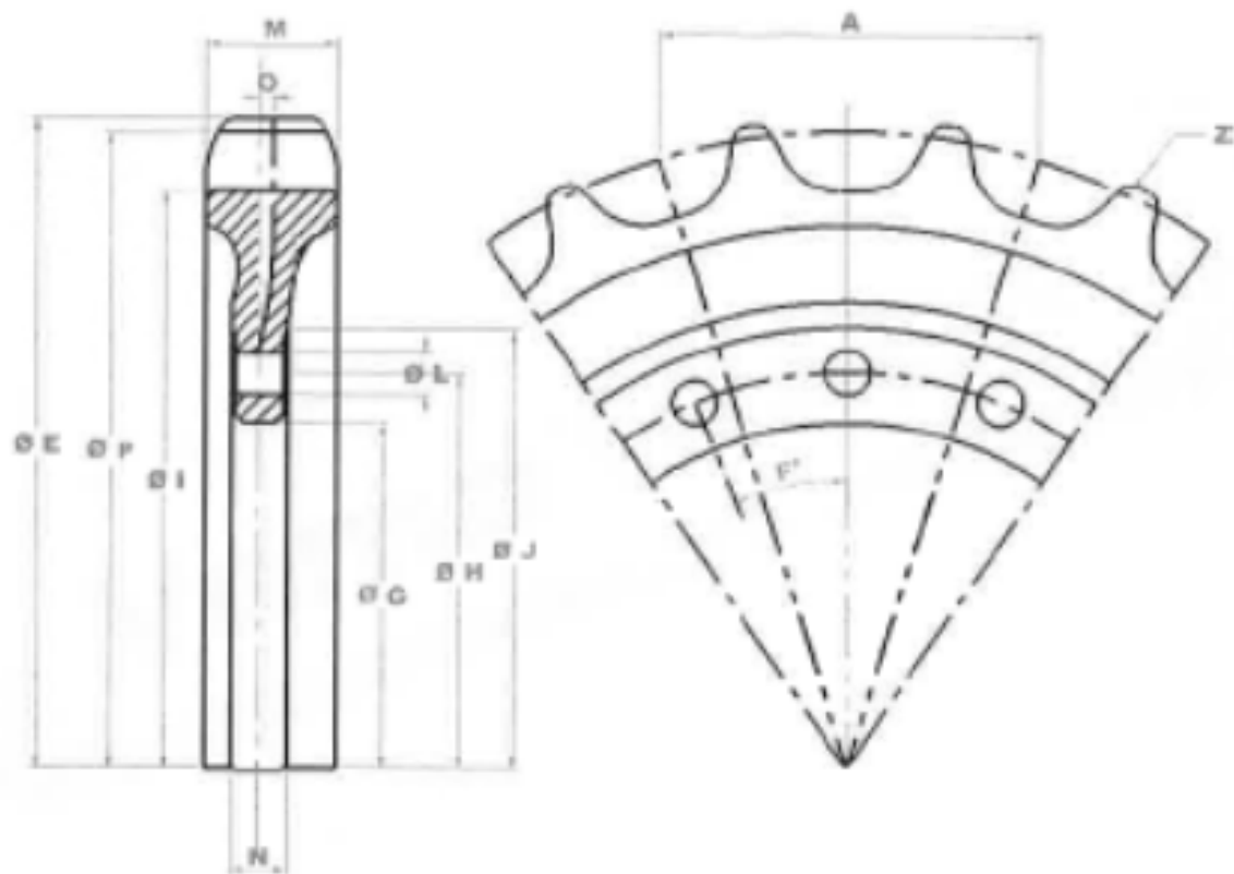
102 Sprocket
