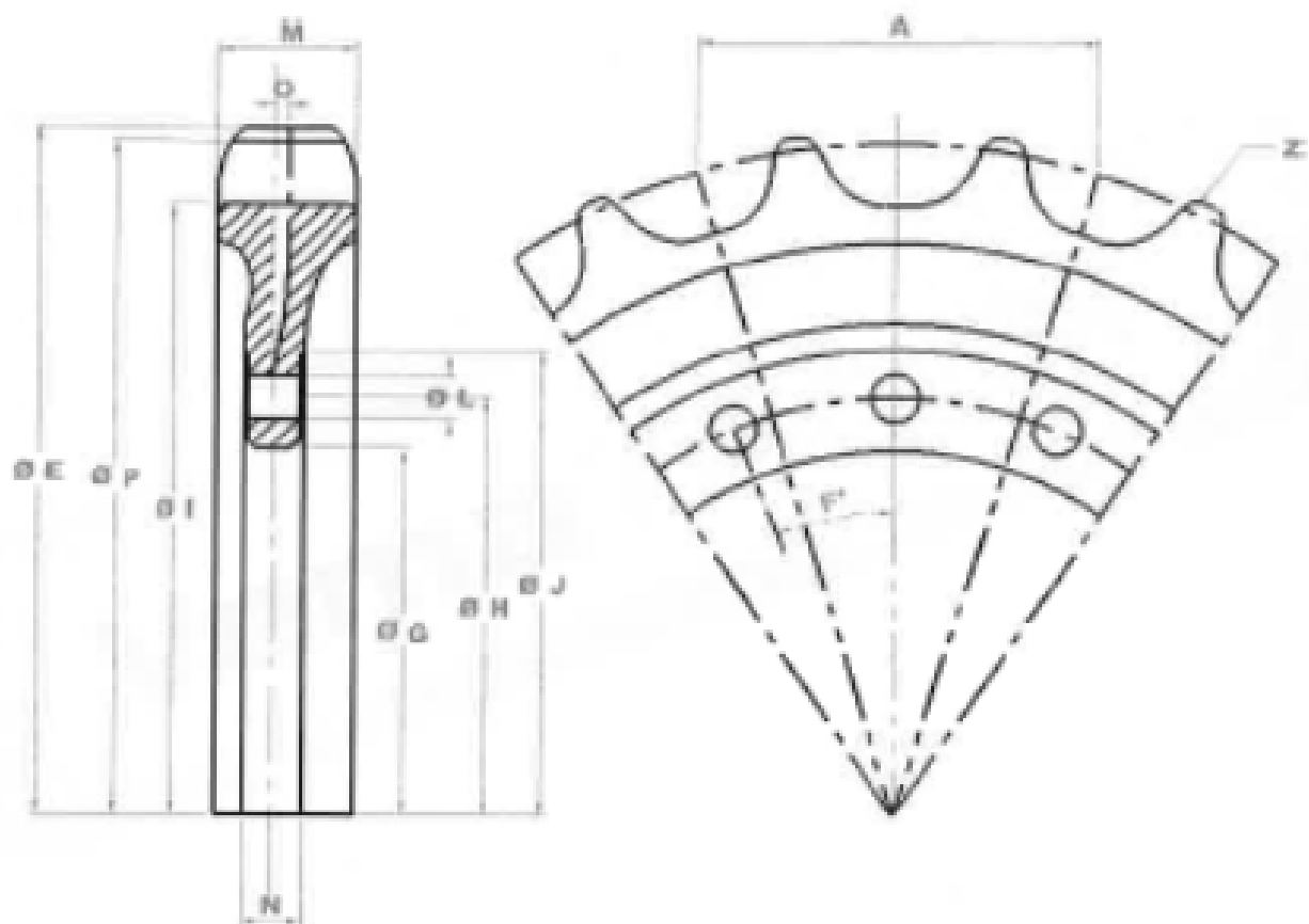
I02 Sprocket
