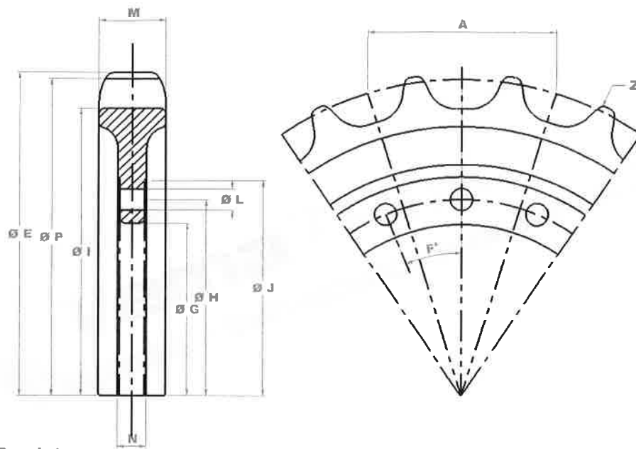
I01 Sprocket
