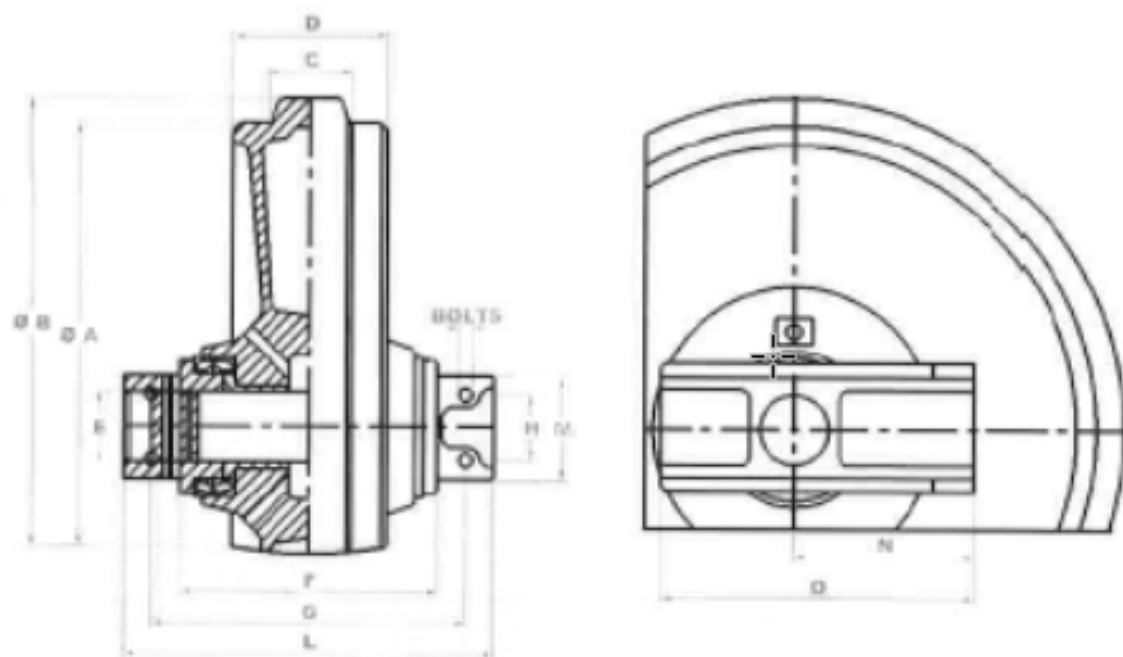
J01 idler
